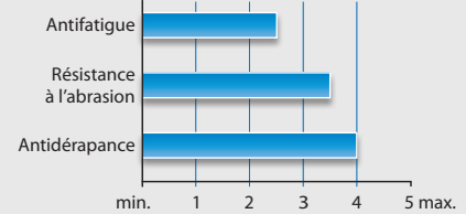
Brosses + jonctions
